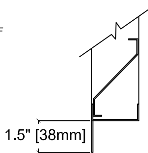
Optional Flange
